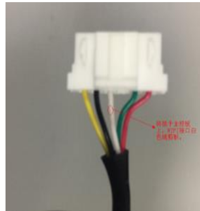
Перерезать белый провод на клемной колодке WiFi модуля
