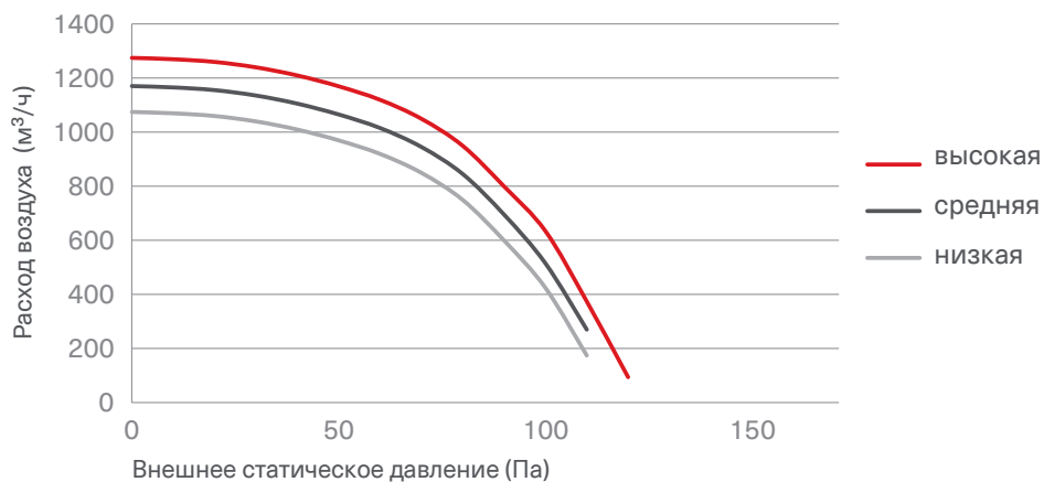
SAD18D3-A
