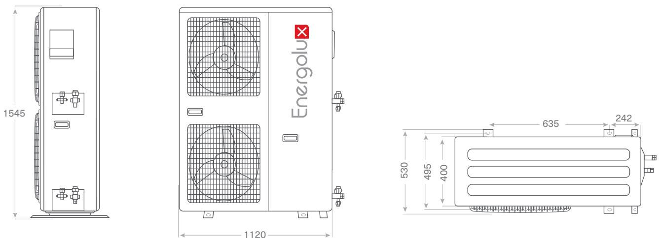
SAU80/100U3-A
