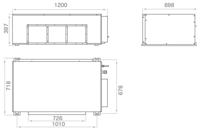
SAD80D3-A, SAD100D3-A
