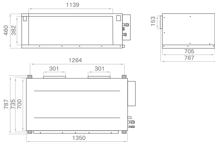
SAD80D3-A, SAD100D3-A
