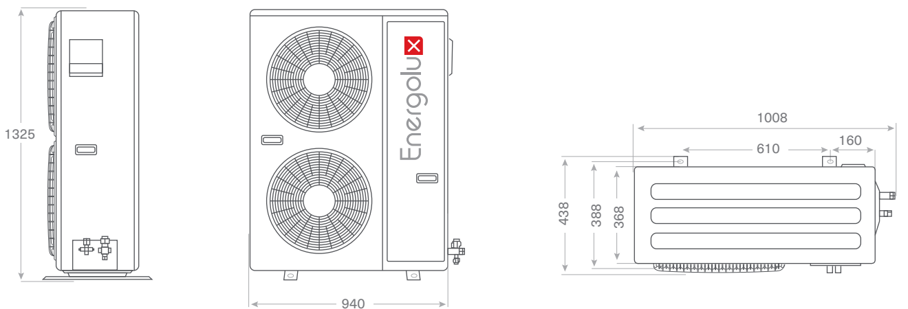
SAU80/100U3-A
