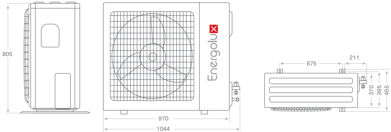
SAU48/60U3-A
