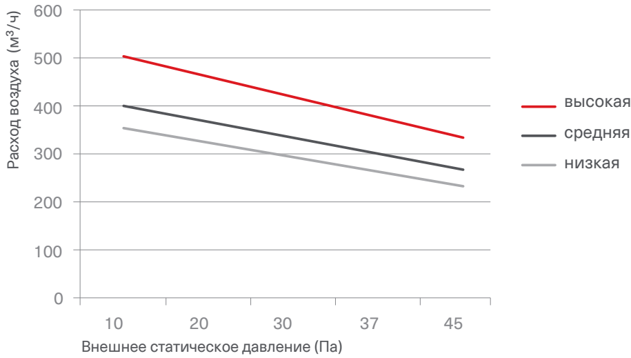
SAD12M1-A1
