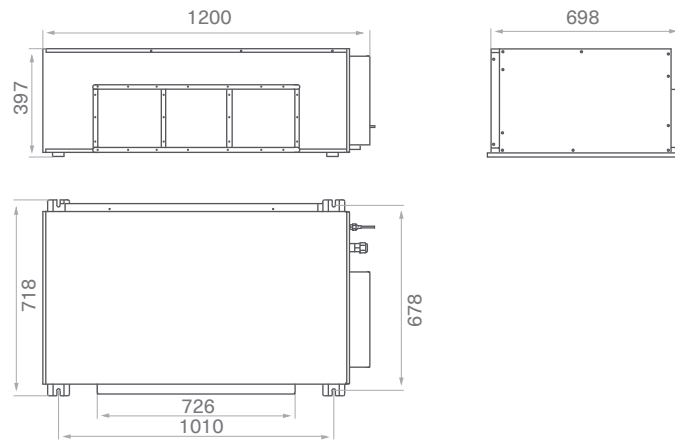
SAD80D3-A, SAD100D3-A
