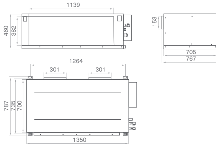
SAD80D3-A, SAD100D3-A
